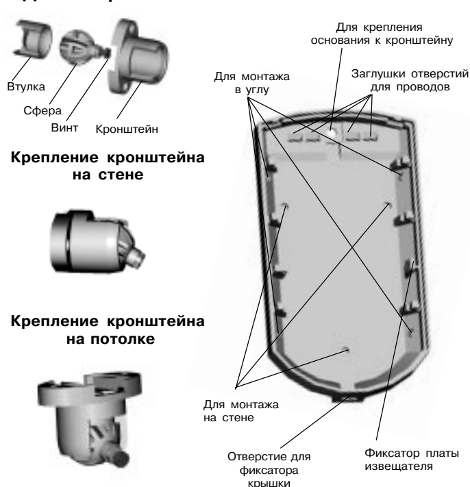
Рис. 2. Основание извещателя и кронштейн
