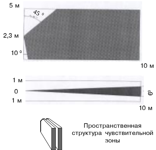
Рис. 1. Диаграмма зоны обнаружения
