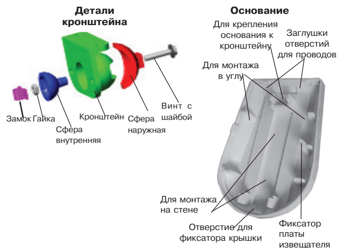
Крепление кронштейна на стене
