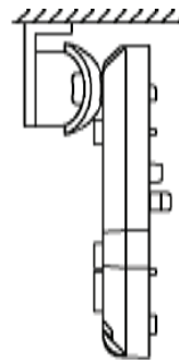
Рисунок 2 - Основание извещателя и кронштейн
