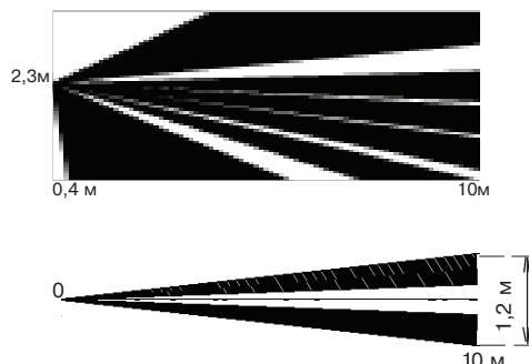
Рисунок 1 - Диаграмма зоны обнаружения
