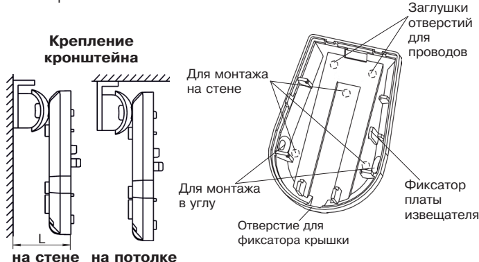
Рисунок 2 – Основание извещателя и кронштейн
