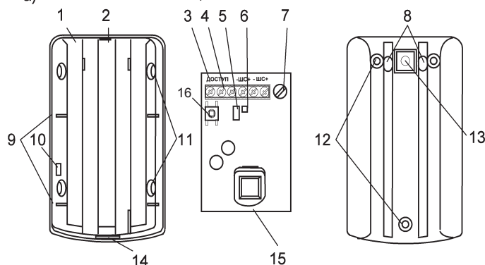
Рисунок 2 – Основание с печатной платой а) основание вид сверху; б) печатная плата; в) обратная сторона основания.
