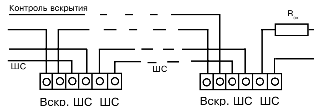
а) параллельно оконечному элементу (режим КЗ)
