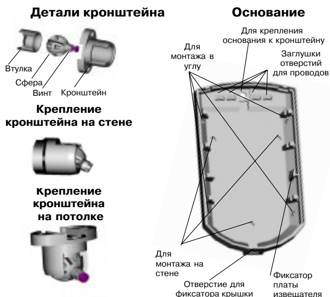
Рис. 2. Основание извещателя и кронштейн
