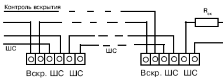
а) параллельно оконечному элементу (режим КЗ)
