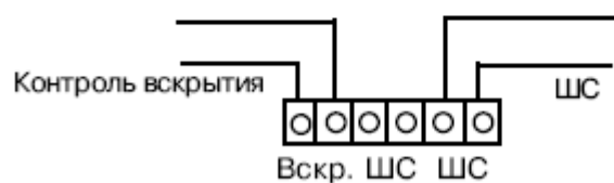
б) вместо выносного элемента (режим РАЗР)
