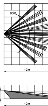
Рисунок 1 — Диаграмма зоны обнаружения
