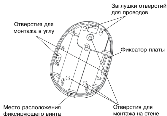
Рисунок 2 – Основание извещателя
