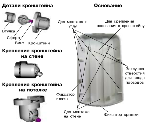
Рис. 2. Основание извещателя и кронштейн
