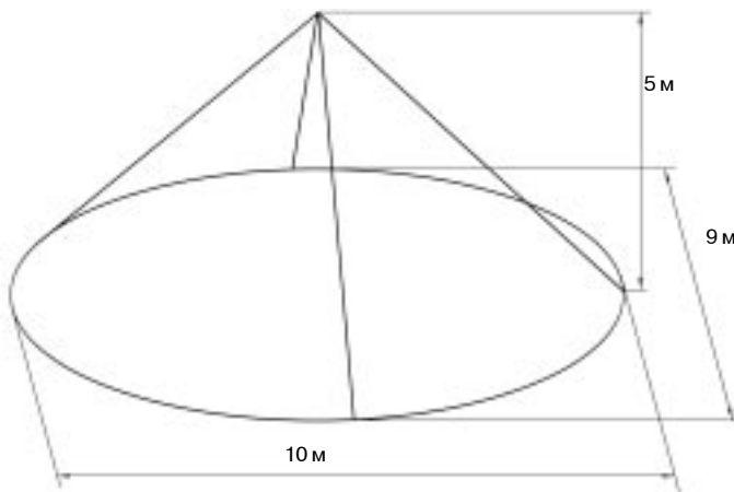
Рис.1 Диаграмма зоны обнаружения
