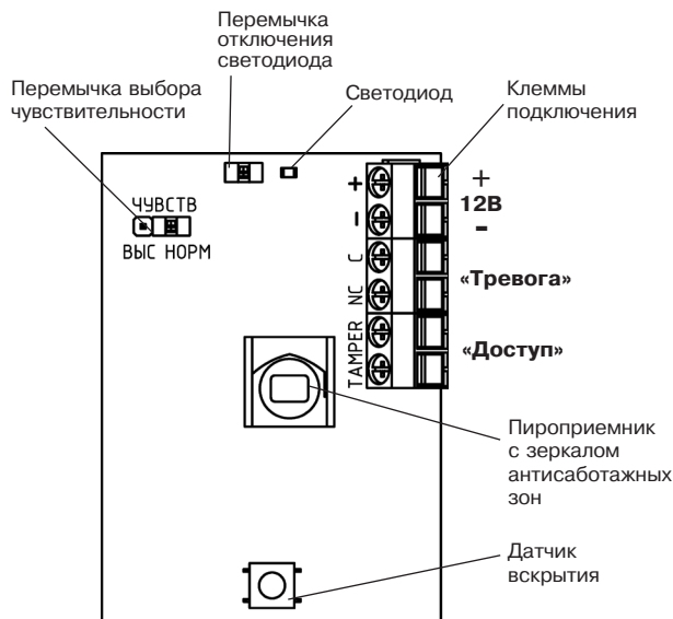
Рисунок 5 – Печатная плата
