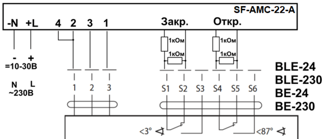
Схема подключения привода с двумя входами
