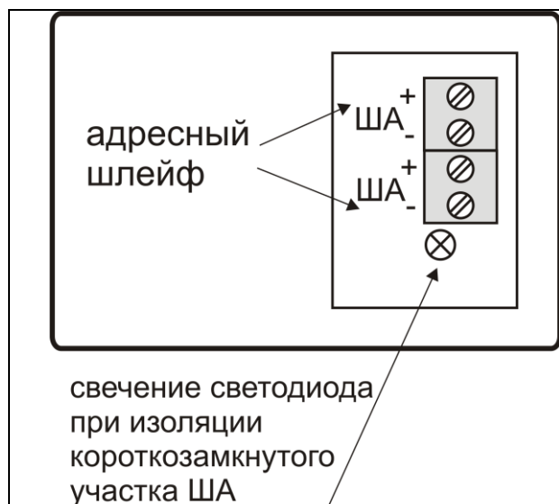
Назначение контактов Исп. 1, Исп. 2
