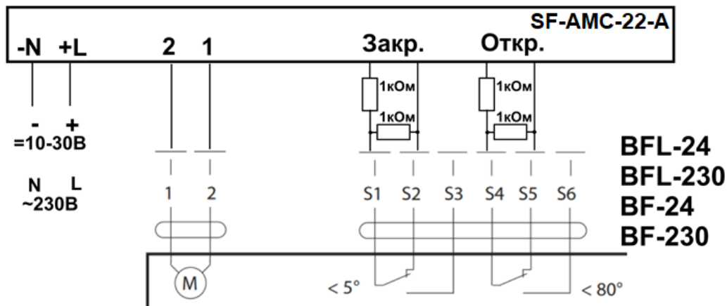
Примеры подключения электроприводов BELIMO
