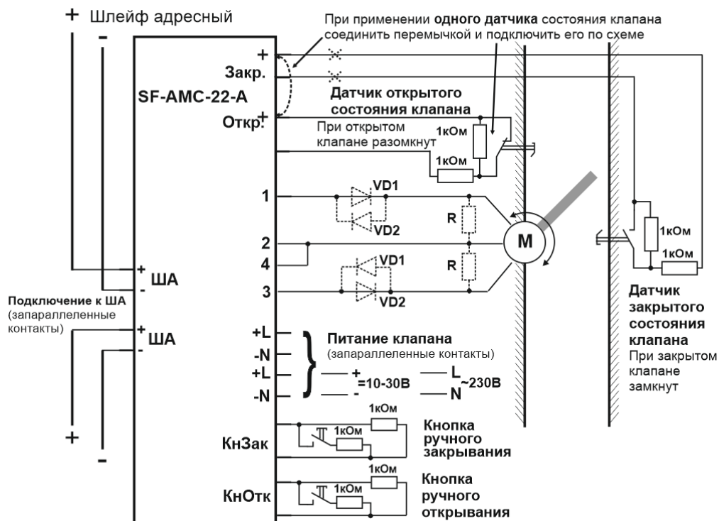
Схема подключения привода с двумя входами
