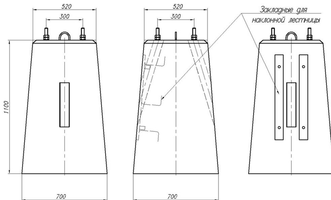
Рис. 2. Габаритные размеры фундамента, положение труб и закладных для лестницы.
