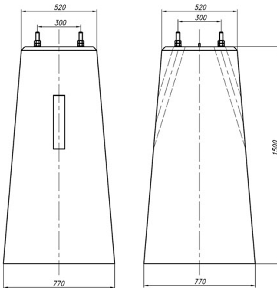
Рис. 2. Габаритные размеры фундамента и положение труб.
