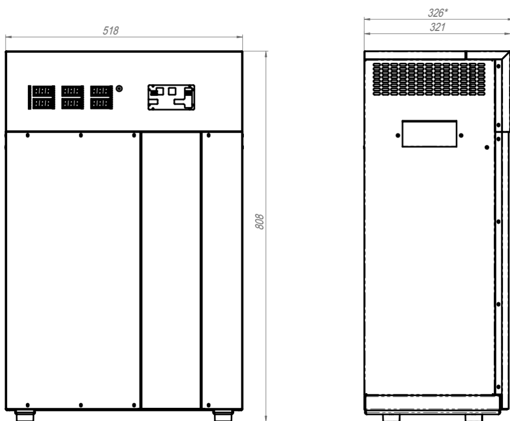
Рисунок 5. Габаритные размеры стабилизаторов Герц на 80А
