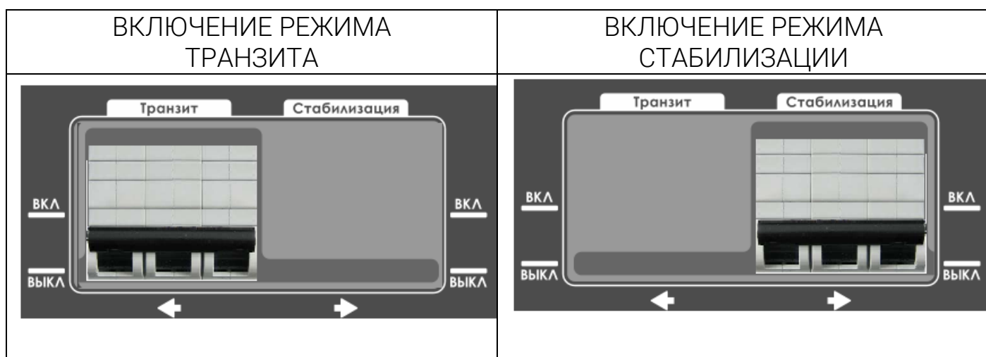
Рисунок 9. Положение тумблера автоматического выключателя при выборе режима работы
