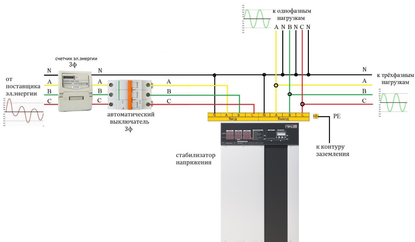
Рисунок 6. Схема подключения стабилизатора к трёхфазной сети
