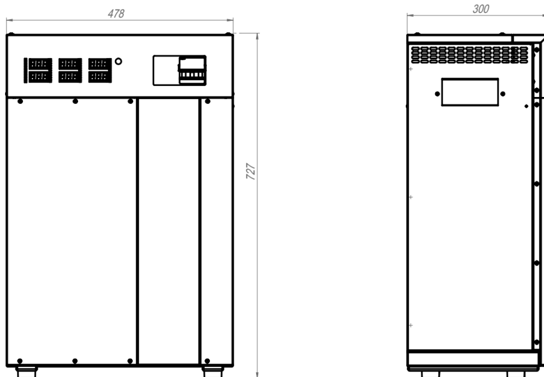
Рисунок 4. Габаритные размеры стабилизаторов Герц на 25-63А
