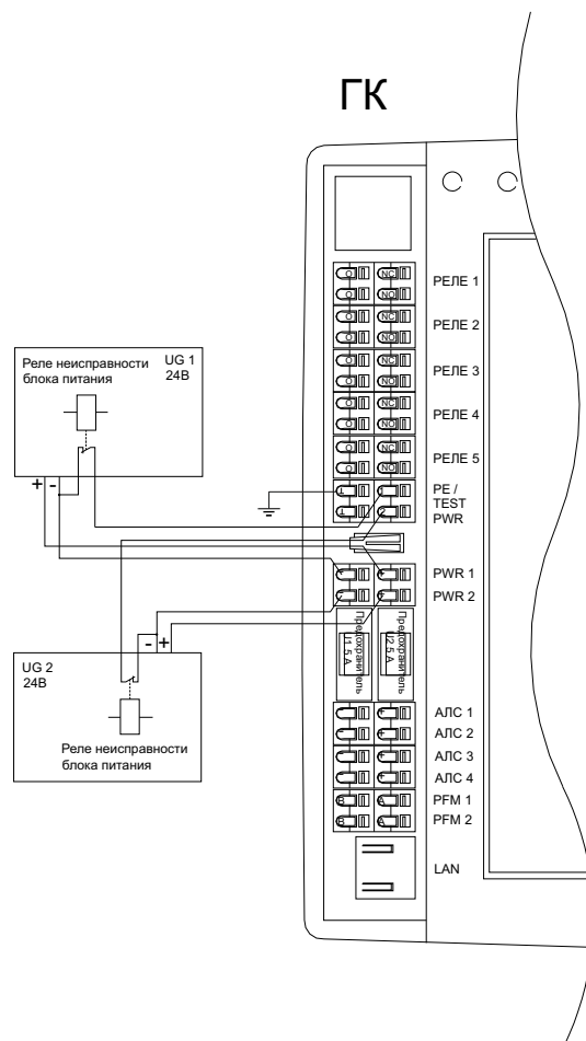
Рисунок В.1 – Схема подключения питания I К исп.3
