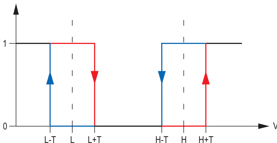
Рис. 11. Способ работы аналогового входа. 0 – отсутствие нарушения. 1 – нарушение.
