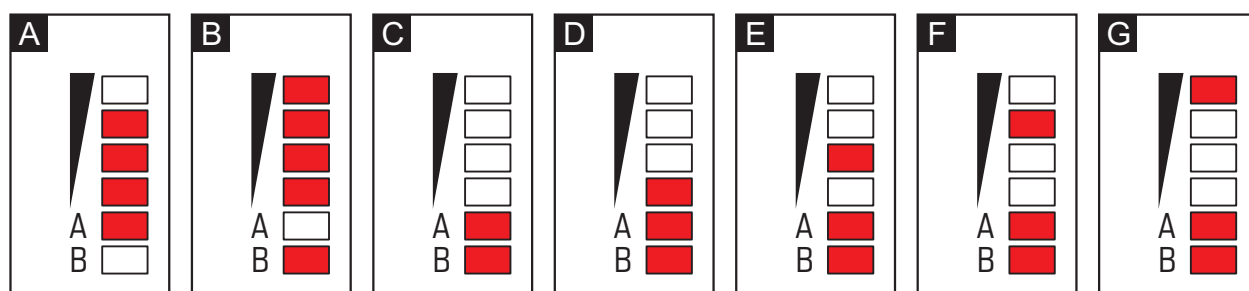
Рис. 3. Примеры светодиодной индикации. Пример А (светодиод А мигает, остальные светодиоды горят) – осуществляется GPRS-передача; уровень сигнала: 3. Пример В (светодиод В мигает, остальные светодиоды горят) – отправляется SMS-сообщение или модуль звонит (тест связи CLIP); уровень сигнала: 4. Пример С (светодиоды мигают) – подключение к GSM-сети.
