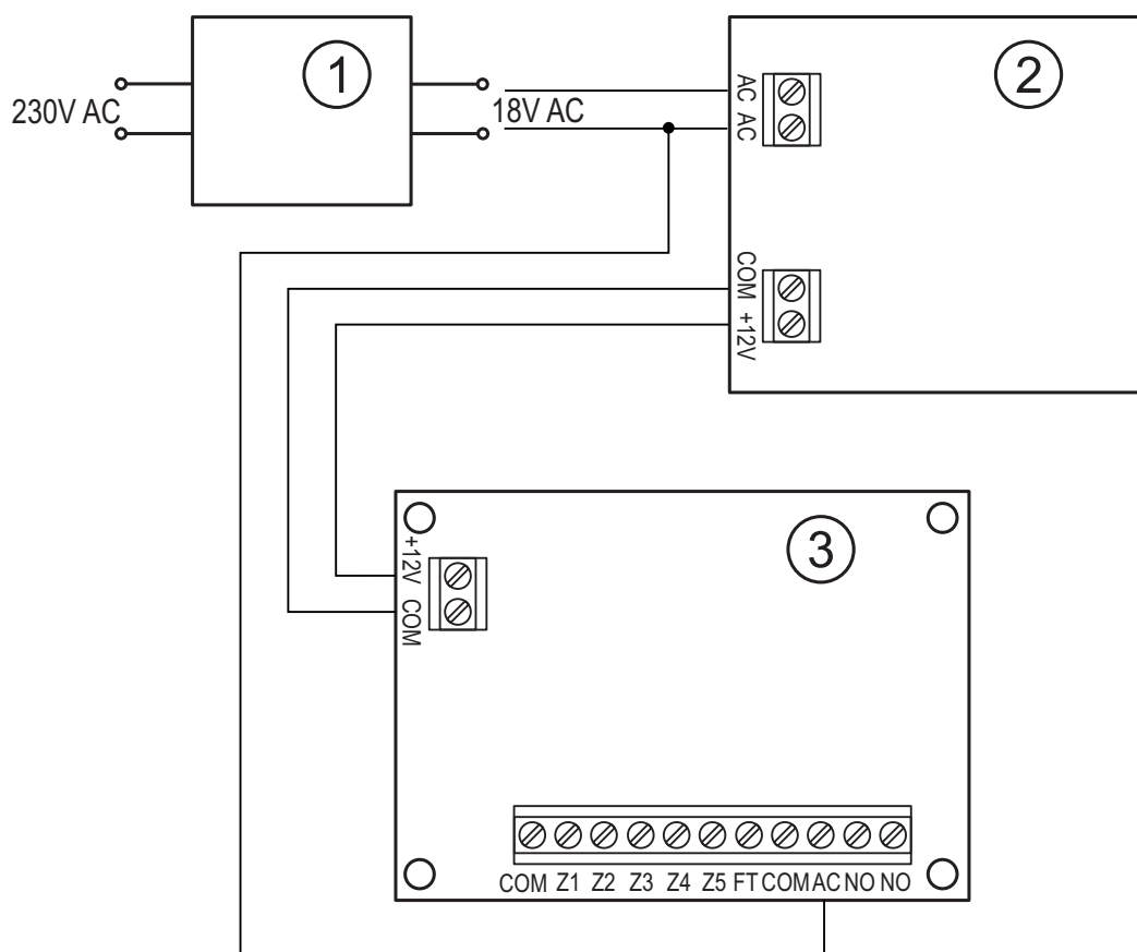
Рис. 4. Пример подключения питания и шлейфа контроля переменного напряжения в модуле GPRS-T2. 1 – трансформатор. 2 – блок питания. 3 – модуль GPRS-T2.
