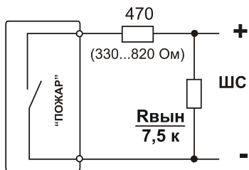
Рис. 6. Организация двухпорогового шлейфа пожарной сигнализации
