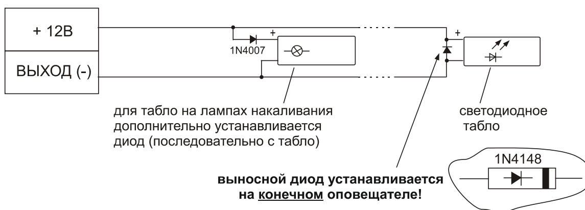
Рис. 9. Схема подключения нескольких световых табло
