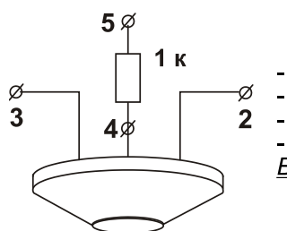
Рис. 5. Организация двухпорогового шлейфа пожарной сигнализации
