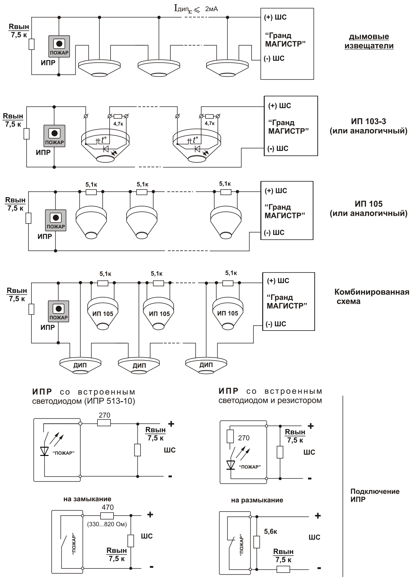
Рис. 7. Организация однопорогового шлейфа пожарной сигнализации
