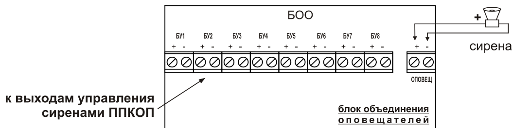
Рис. 10.2. Схема подключения одного звукового оповещателя (сирены) к нескольким приборам "Гранд МАГИСТР"
