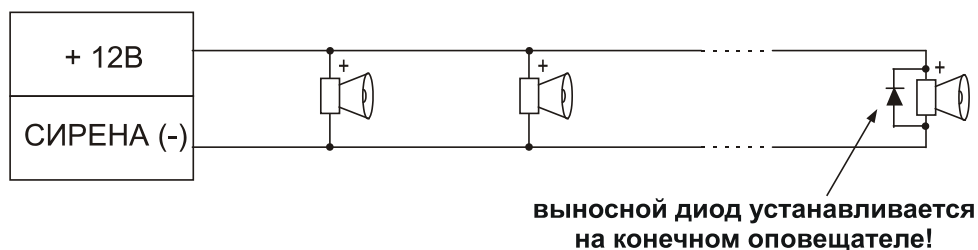
Рис. 10.1. Схема подключения нескольких звуковых оповещателей
