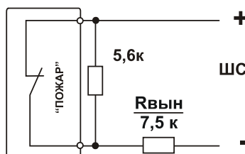
Рис. 6. Организация двухпорогового шлейфа пожарной сигнализации
