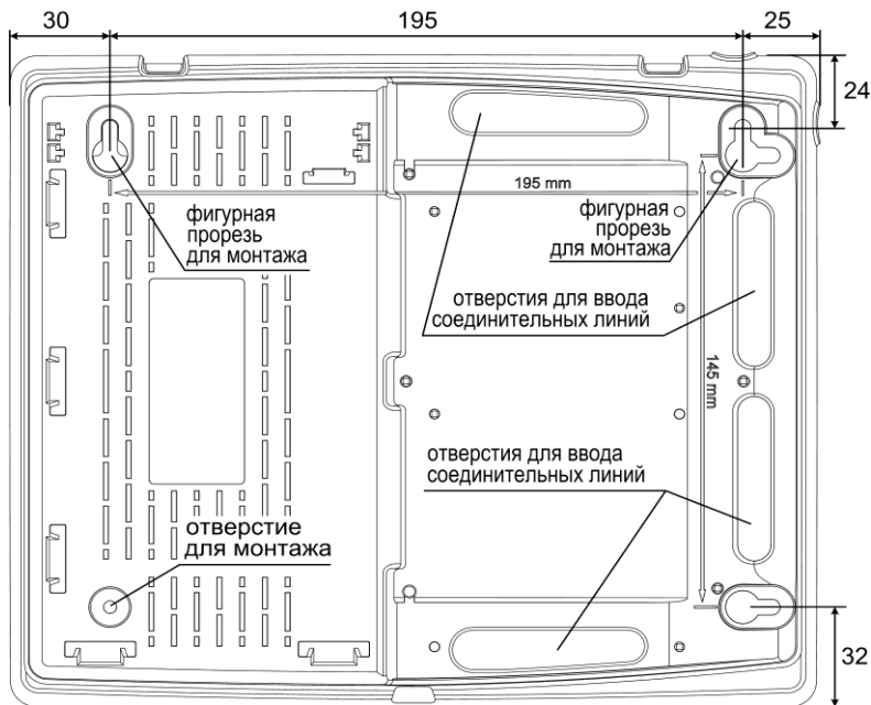
Рис.3 Задняя стенка прибора. Присоединительные размеры
