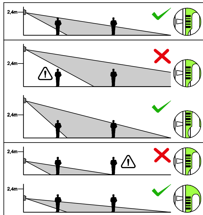
Рис. 3. Влияние высоты монтажа на защищаемую извещателем зону и способ позиционирования пирозлемента по отношению к линзе с целью оптимальной установки.
