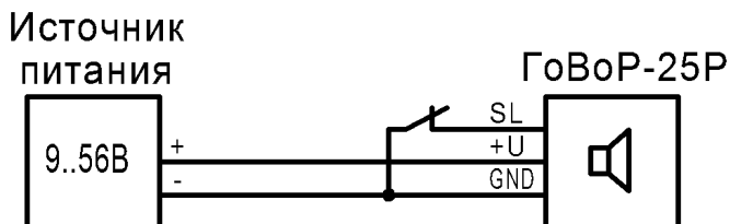
Рис. Б.3 Схема подключения ГоВоР-25Р при выборе сообщений.
