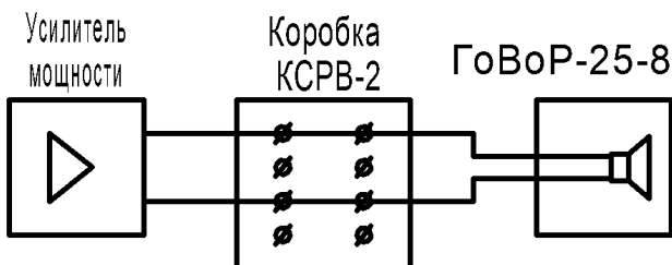
Рис. Б.1 Схема подключения ГоВоР-25Т, ГоВоР-25-8.
