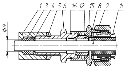
з) монтаж бронированным кабелем в металлорукаве в кабельном вводе КВМ
