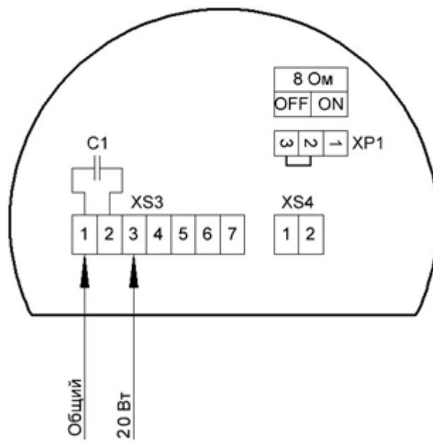
Рисунок Б2 – Схема подключения ГВР-Exd-20
