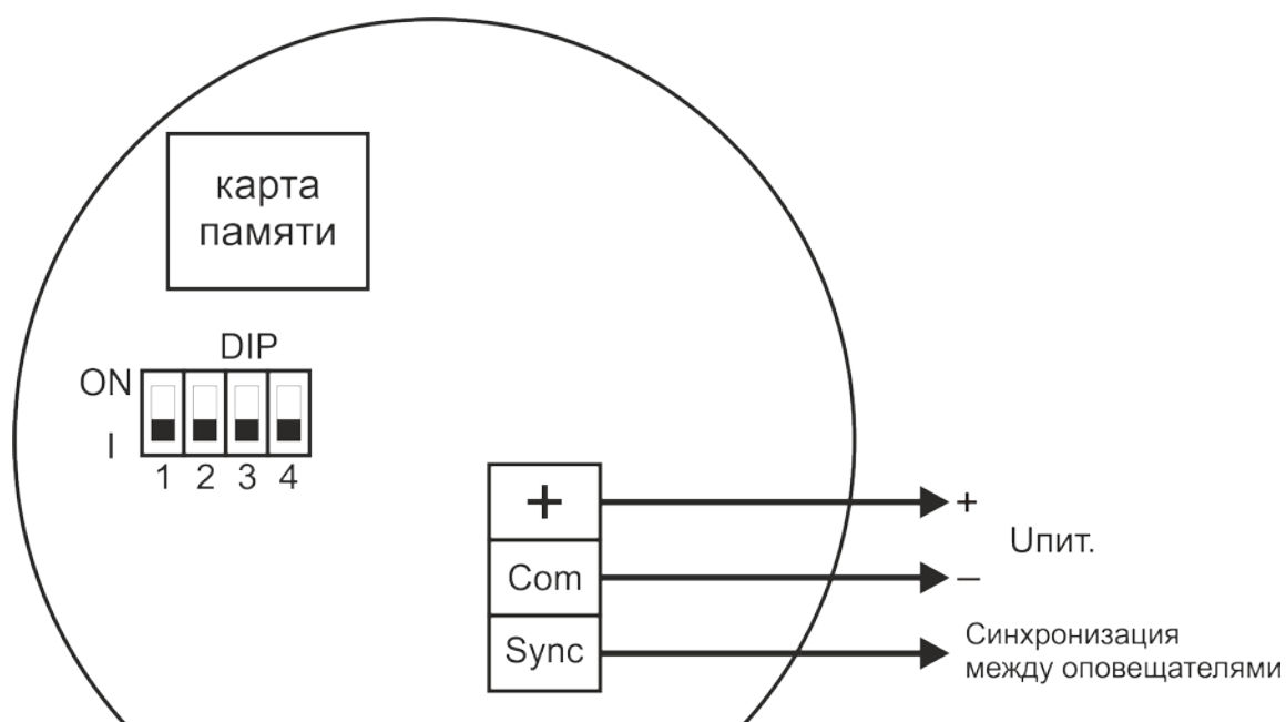
Рис. Б6 – Схема подключения РЗОП-Exd-10, РЗОП-Exd-20, РЗОП-Exd-30, РЗОП-Exd-50
