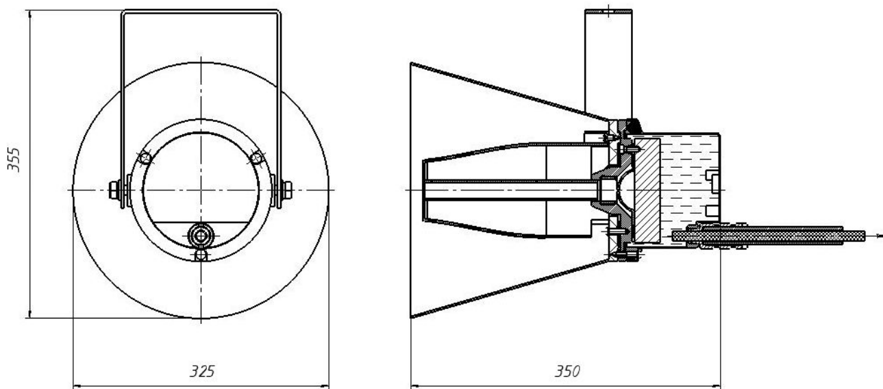
Рисунок 4 – Габаритные размеры оповещателя «LPA- 50Exm»
