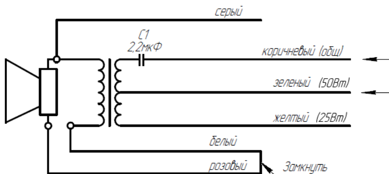
Рисунок 8 – Схема подключения LPA-Exm50
