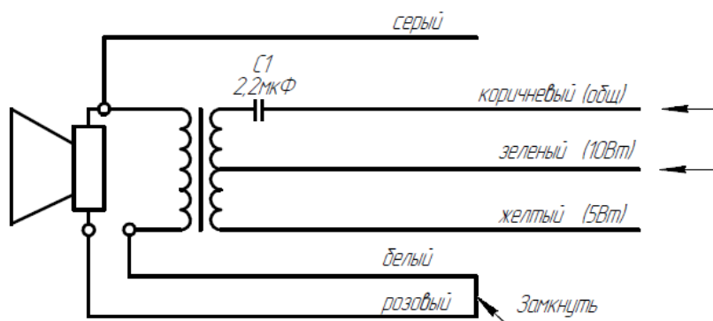
Рисунок 5. Схема подключения LPA-Exm10
