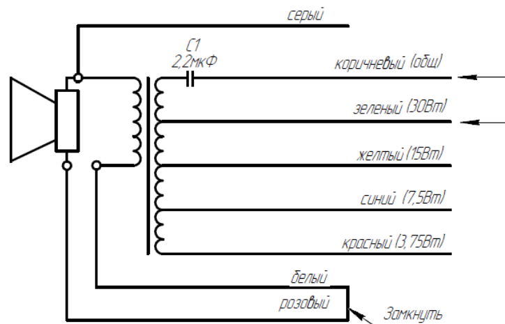
Рисунок 7 – Схема подключения LPA-Exm30
