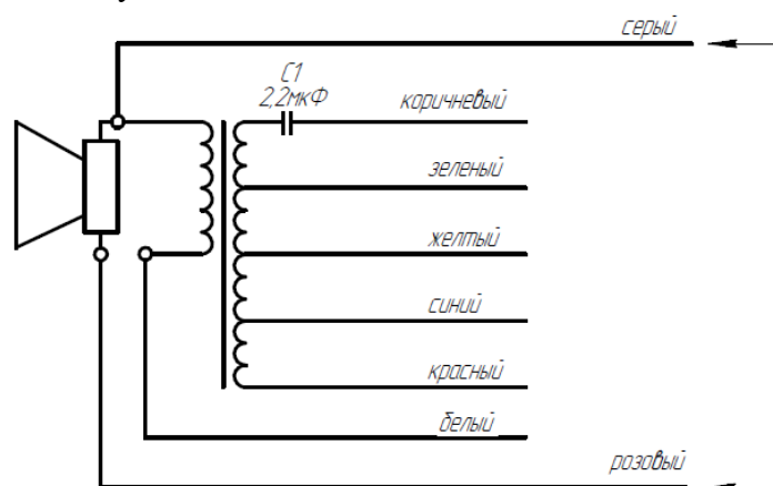
Рисунок 8 – Схема подключения LPA-Exm50
