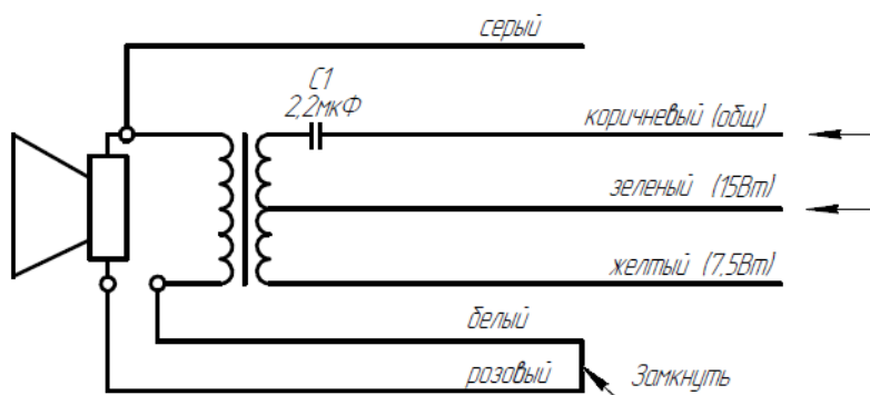
Рисунок 6. Схема подключения LPA-Exm15
