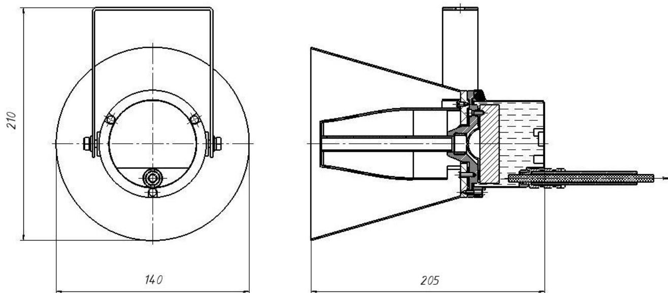
Рисунок 1 – Габаритные размеры оповещателя «LPA-10Exm»
