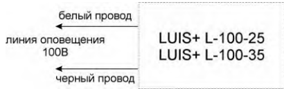
Рисунок 1. Схема подключения
