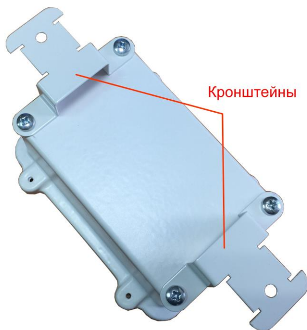
Рис. 5.1. Кронштейны устройства
