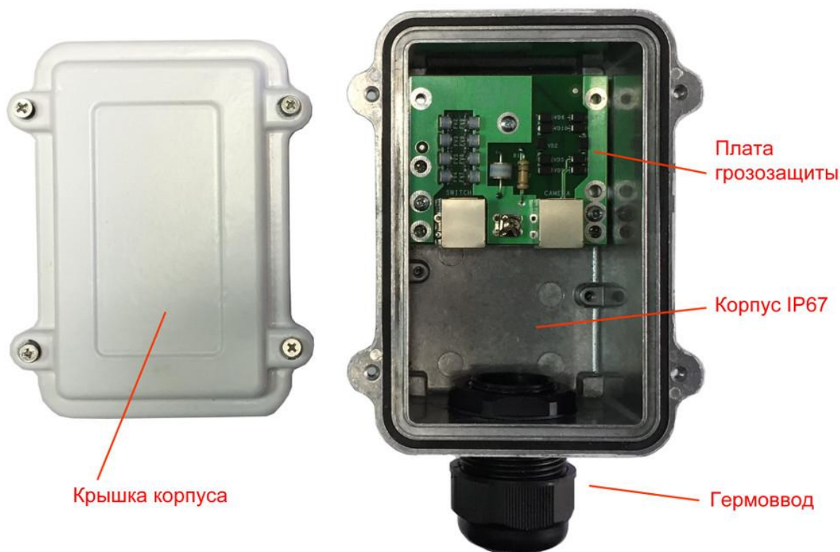
Рис. 2-1. TFortis SG-Cam – внешний вид
