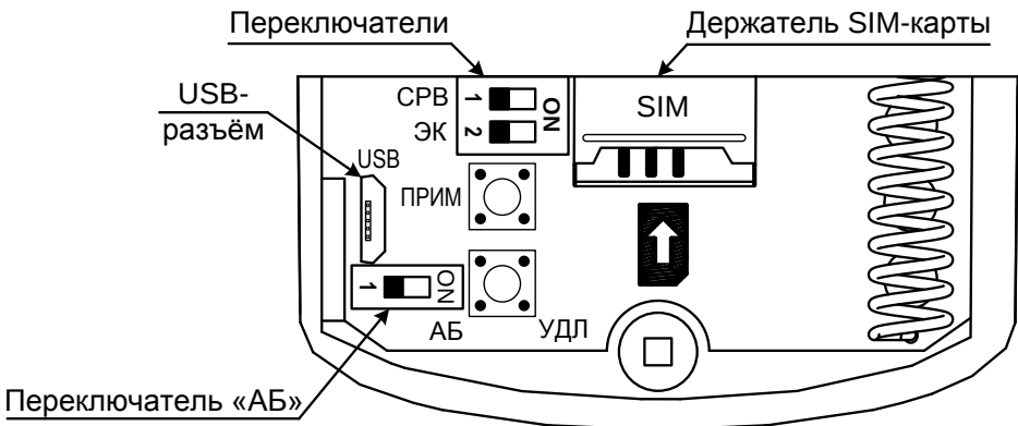
Рис.А2. Внешний вид платы прибора «GSM РОЗЕТКА ВЕКТОР» (видимая часть). Вид на разъемы и органы управления прибора
