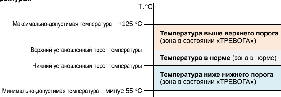
Рис.2. Алгоритм работы прибора в режиме автоматического информирования о выходе температуры за установленные пороги
