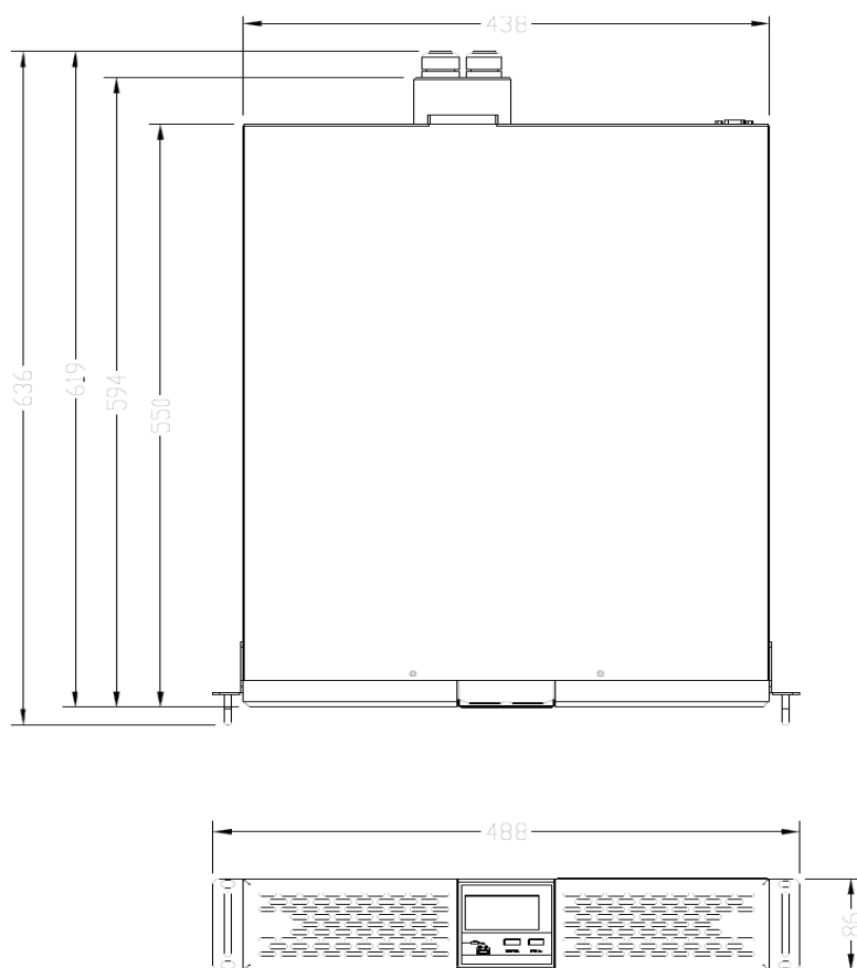
Габаритные размеры
