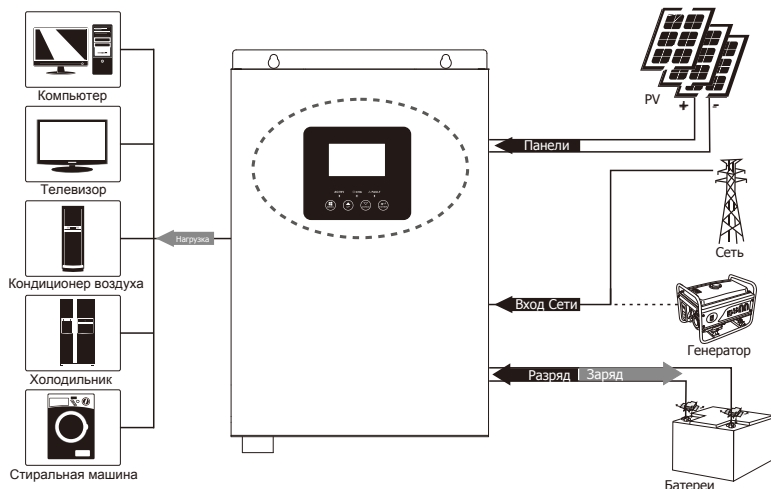
Рисунок 1. Гибридная система электропитания
