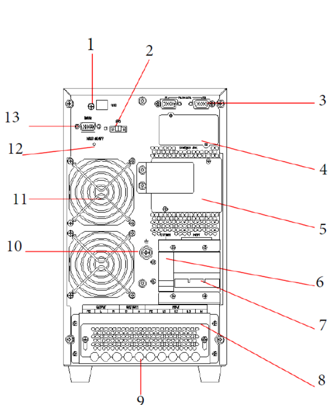
Рис. 1-2 Вид сзади
