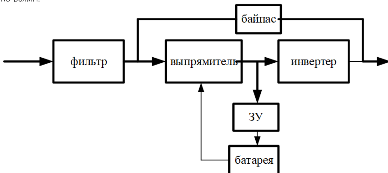
Рис. 3-5 ЭКО режим
