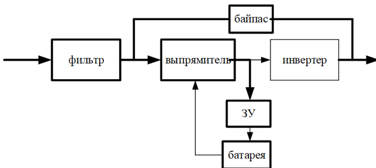
Рис. 3-3 Режим байпаса
