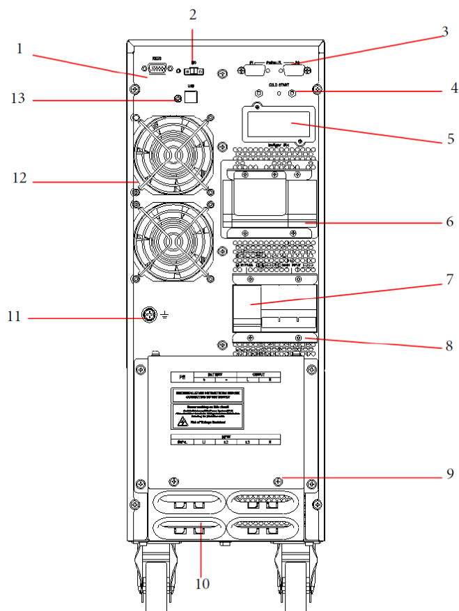
Рис. 1-2 Вид сзади
