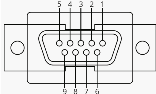
Рис. 7-1 DB9 порт
