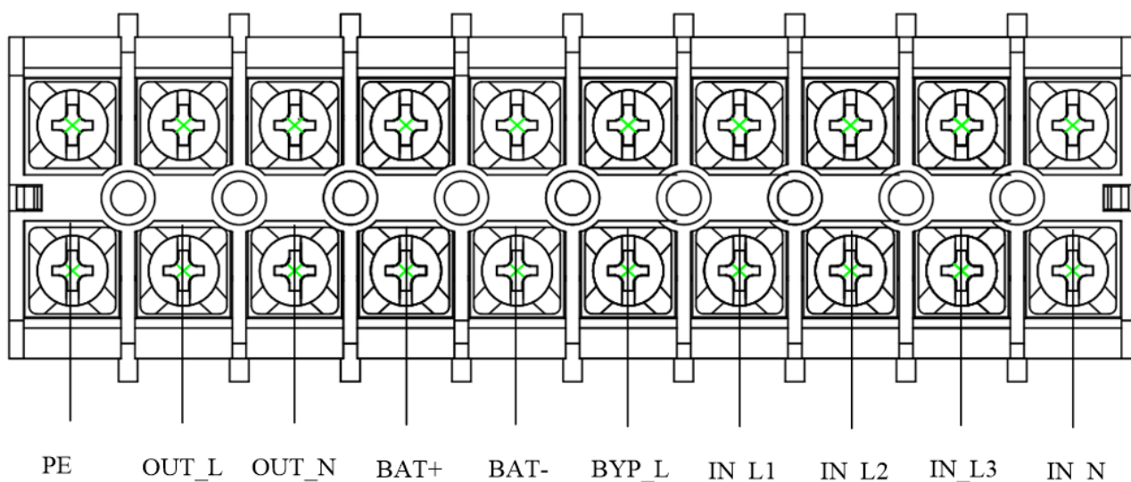
Рис. 4-1 Клеммная колодка 10кВА
