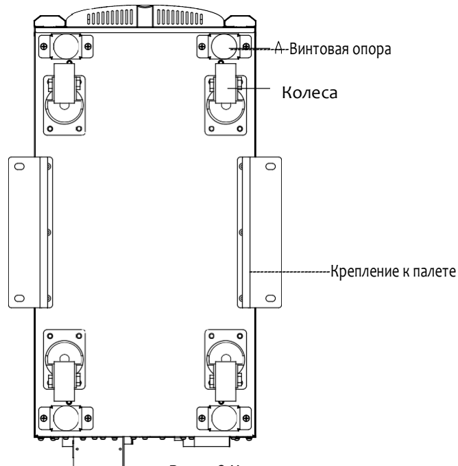
Рис. 2-8 Колеса и опоры.
