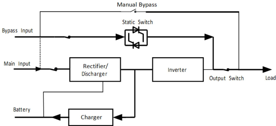
Рис 1-6. ECO режим
