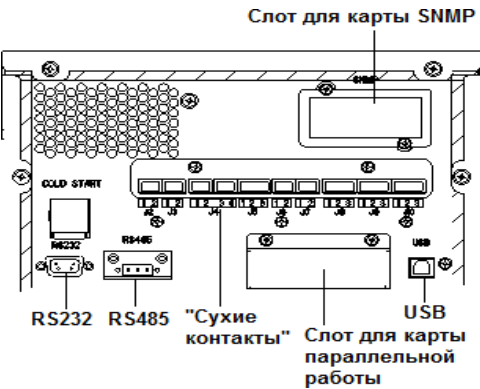
Рис.2-14 Коммуникационные порты
