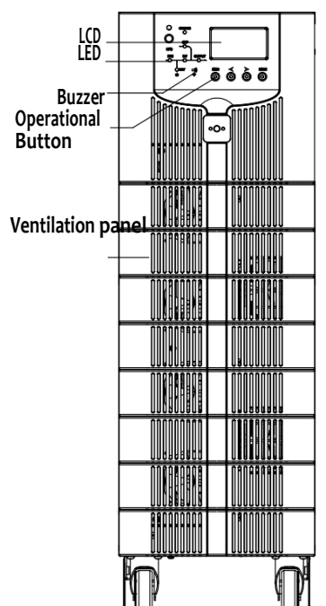
Рис 1-10. 10-30kVA Вид спереди
