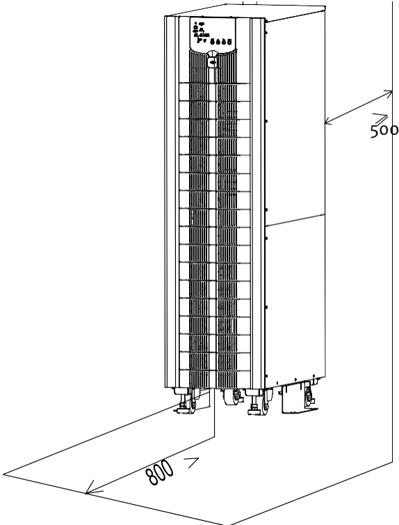
Рис. 2-4.. Минимальное пространство вокруг ИБП
