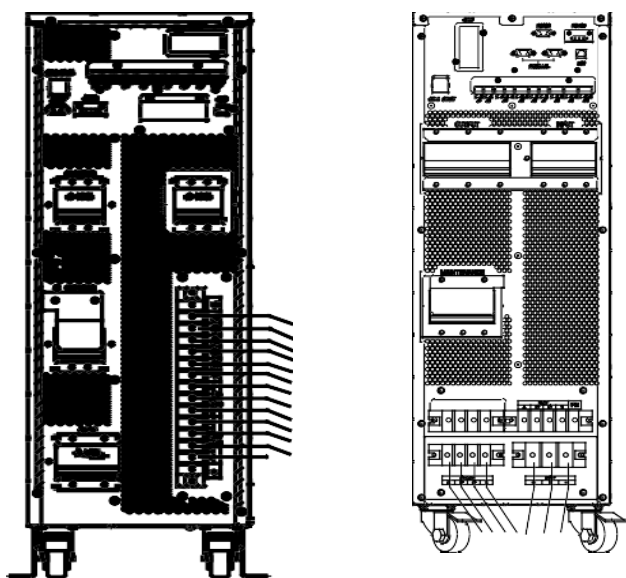
Рис. 2-10. Подключение кабелей.
