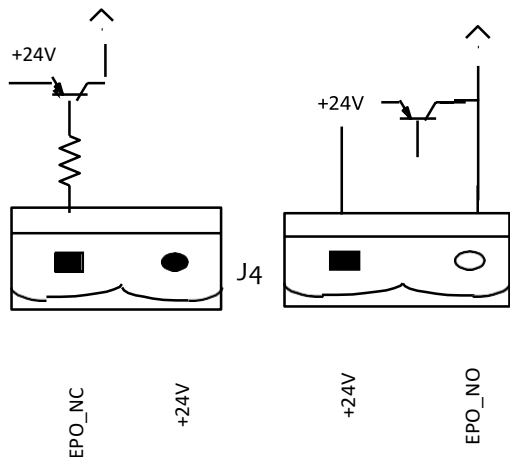
Рис.2-16 Схема разъема системы экстренного отключения (ЕРО)
