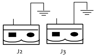
Рис.2-15 Схема разъемов J2 и J3 для датчиков температуры Таблица
