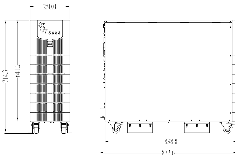
Рис. 2-1-2. Разморо/15 kVA с внутренними батареями
