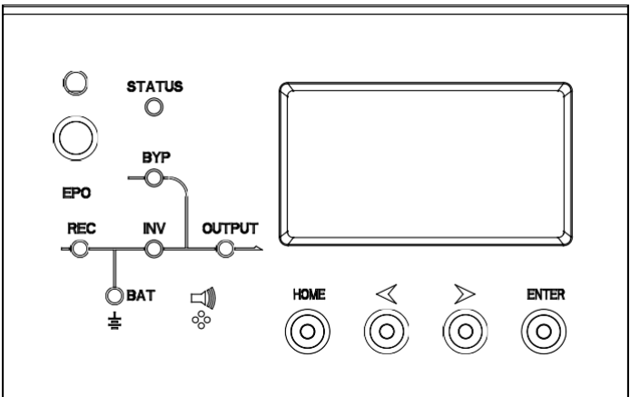
Рис. 3-1. Панель управления
