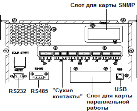
Рис.2-14 Коммуникационные порты
