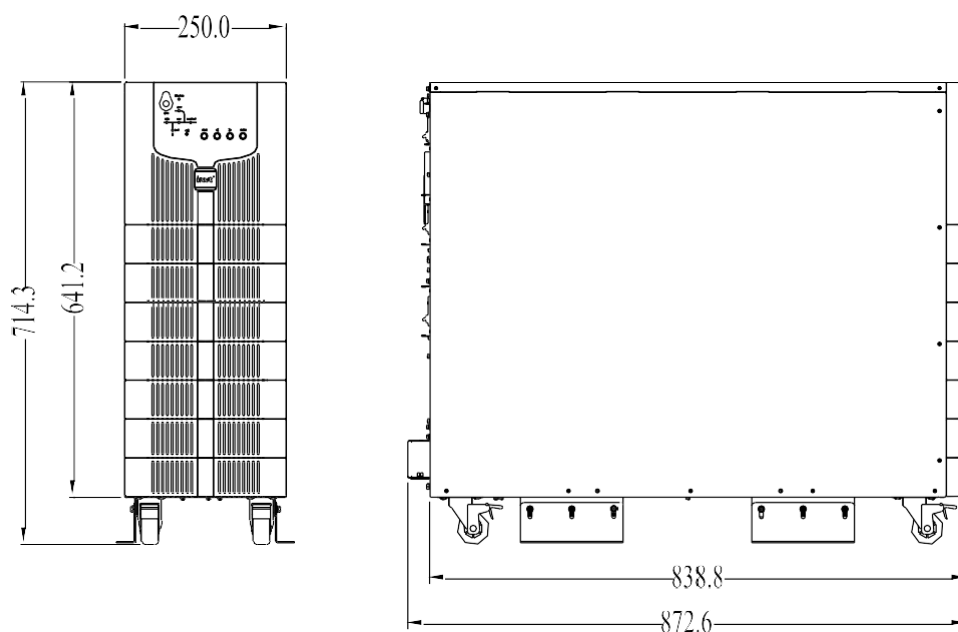
Рис. 2-1-2. Размеры 10/15 kVA с внутренними батареями
