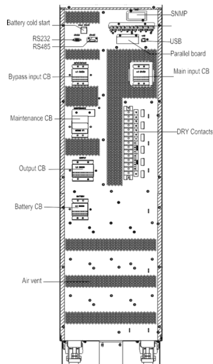
Рис 1-14. 20/30kVA Вид сзади со встроенными батареями
