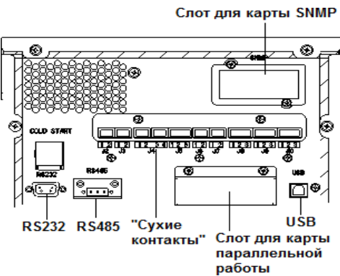
Рис.2-14 Коммуникационные порты
