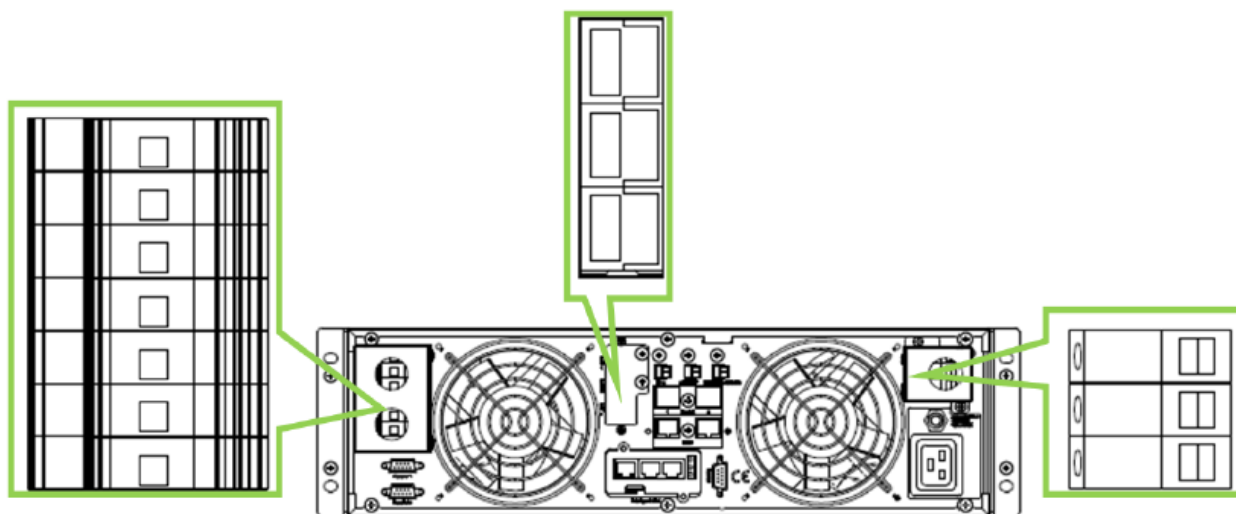
Рис. 3-3 Схема соединений
