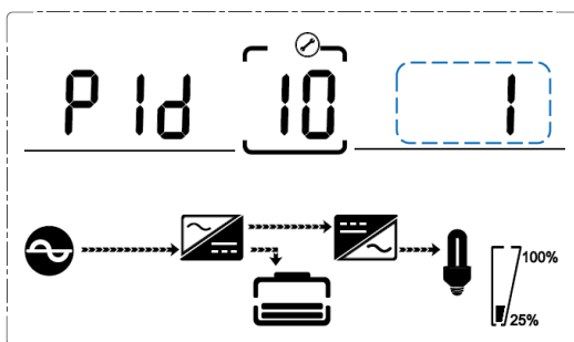
Рис. 4-12 Меню настройки идентификатора при параллельной работе ИБП (Примечание: изображение, выделенное пунктиром, мигает)
