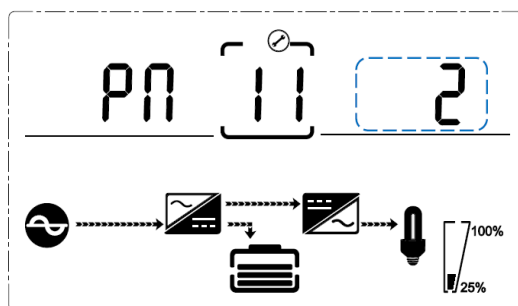
Рис. 4-12 Меню настройки количества резервных модулей (Примечание: изображение, выделенное пунктиром, мигает)
