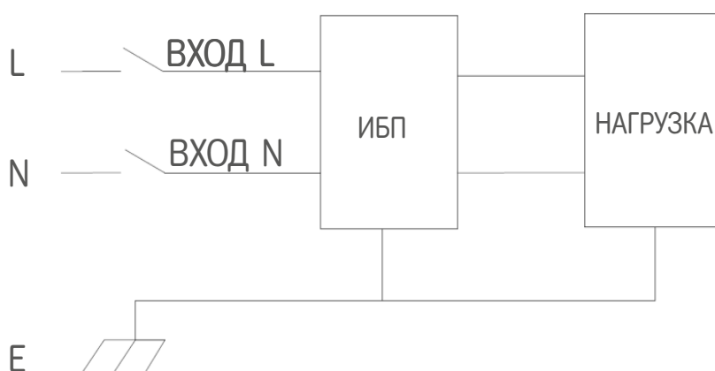
Рис. 3-3 Схема соединения на входе – «одна фаза + земля»
