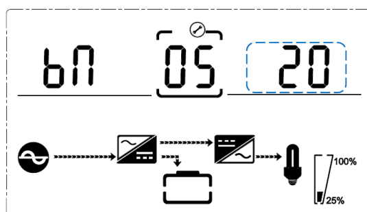
Рис. 4-7 Настройка количества АКБ
