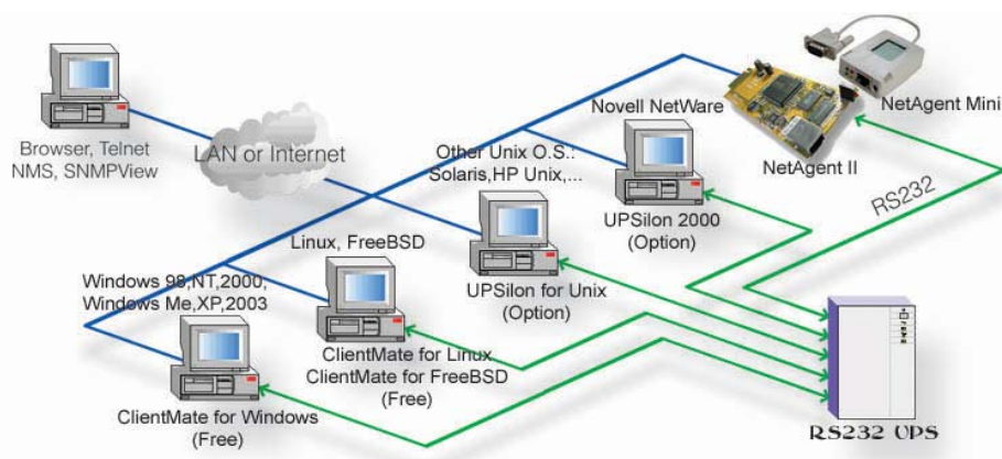
Рис.1. NetAgent подключение программного обеспечения
