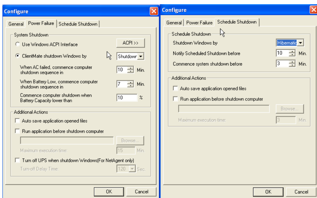
Рис.64 Конфигурация ClientMate
