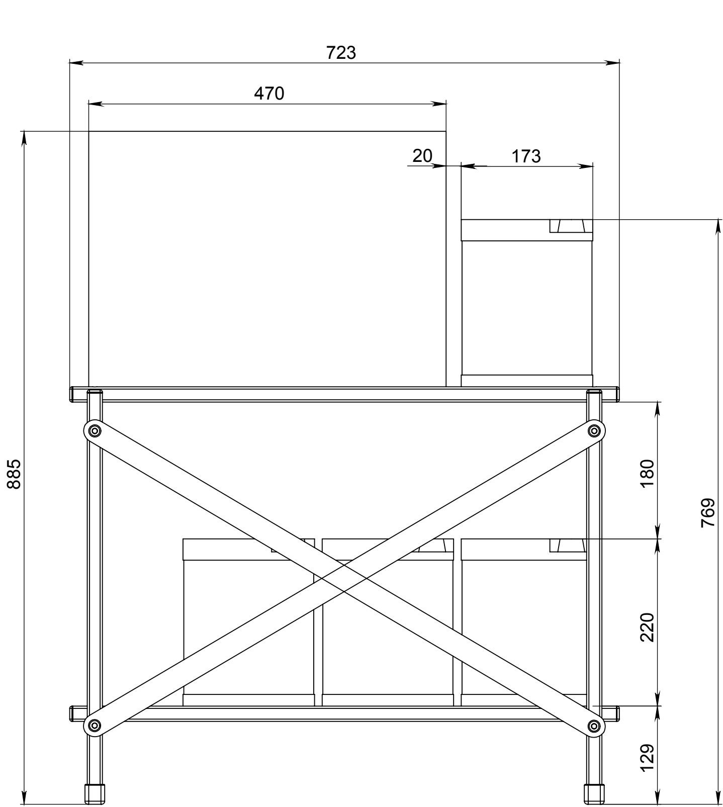
Нагруженный вид
