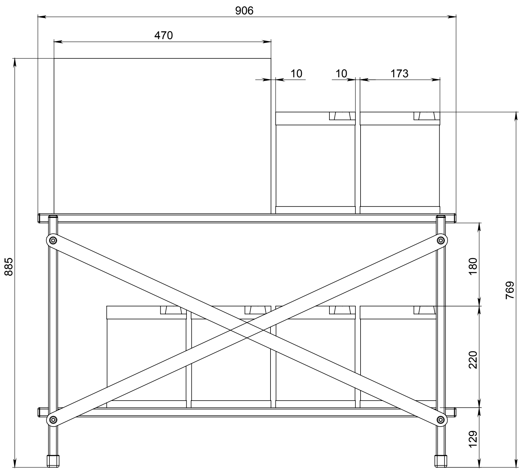
Нагруженный вид
