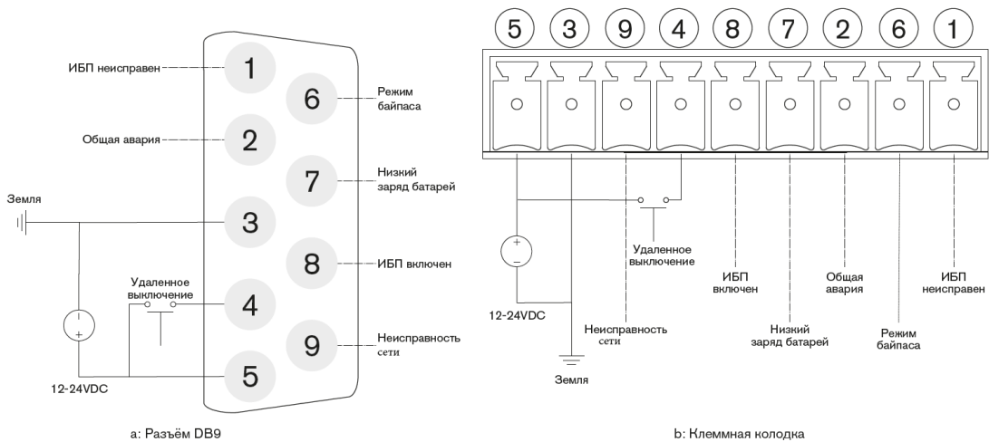
Рис. 9-1 Схема подключения сухих контактов
