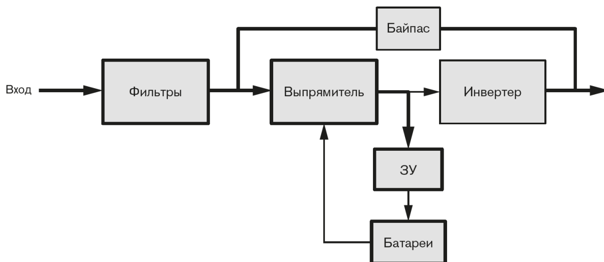
Рис. 3-3 Режим байпаса
