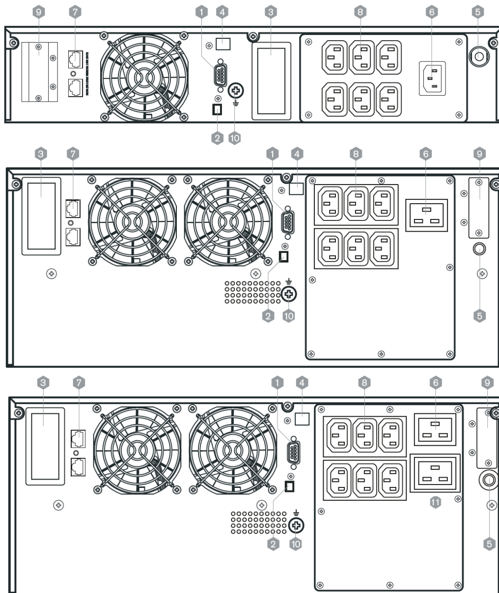
Рис. 1-3 UDC9200S-RT 1-3 кВА
