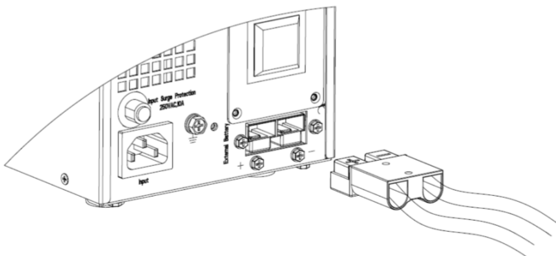
Рис. 4-2 Подключение АКБ
