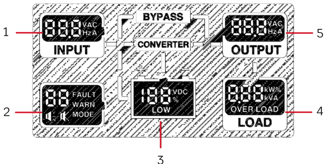
Рис. 5-2 LCD дисплей
