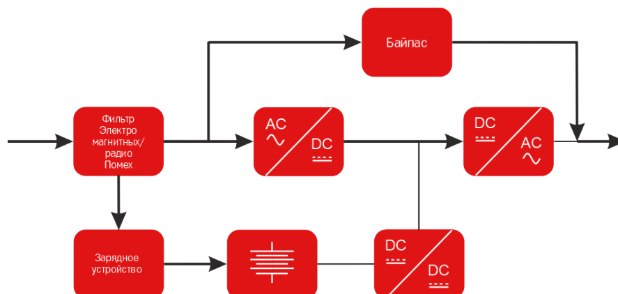
Рис. 3-5 ЭКО режим
