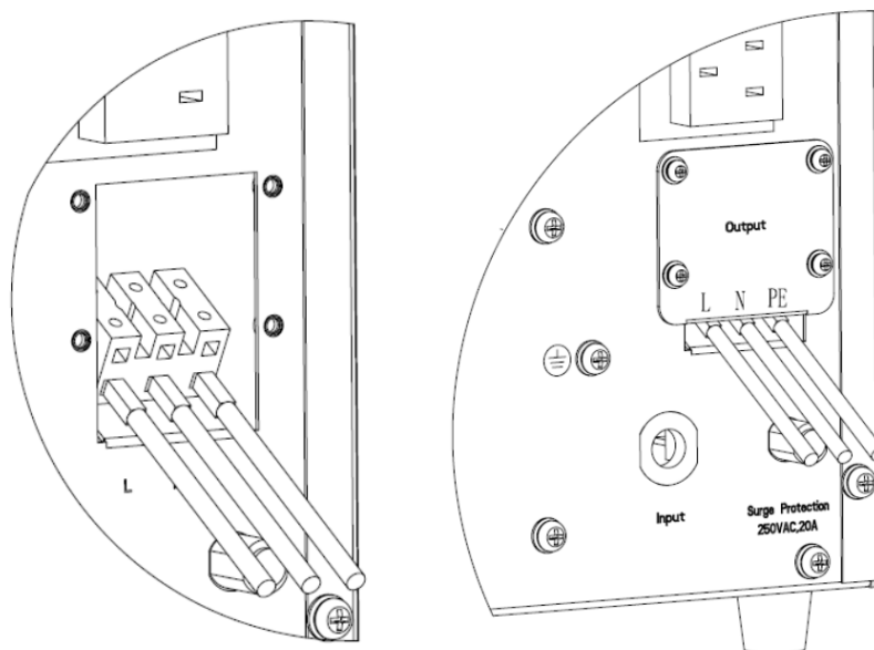
Рис. 4-1 Выходная колодка ИБП 3 кВА
