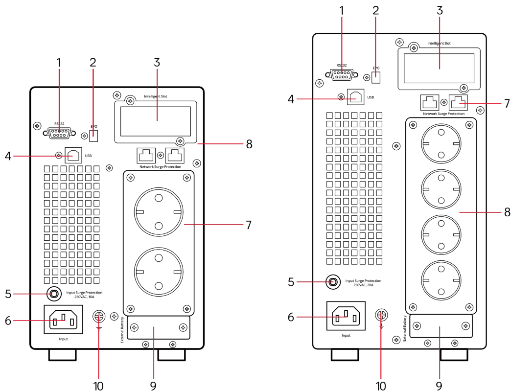
Рис. 1-2 Вид сзади
