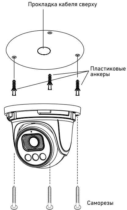
Рис. 3. Монтаж камеры
