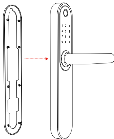
Установите вал и нижний скользящий винт
