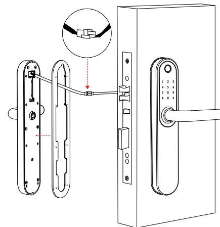
Установка внутренней панели
