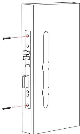
Установите врезную часть и цилиндр
