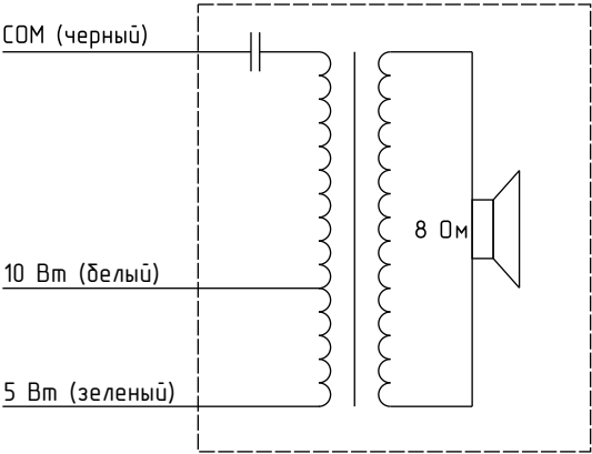
Рисунок 5.1 Принципиальная схема громкоговорителя
