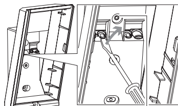
Проводное отверстие
