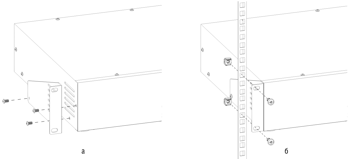
Рисунок 7.1 Установка ИБП в телекоммуникационную стойку или шкаф: а – установка монтажных уголков; б – закрепление ИБП на направляющей при помощи крепёжных комплектов.
