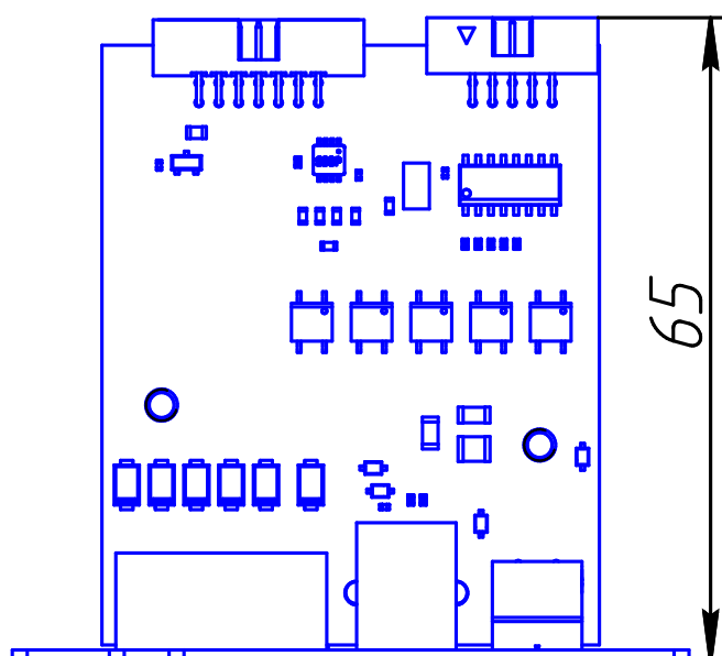
Рисунок 1.2 – Габаритные размеры изделия
