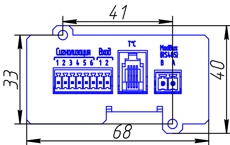
Рисунок 1.1 – Внешний вид изделия
